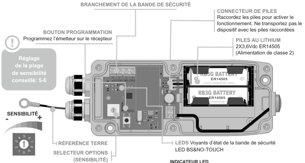
INDICATEUR LED
