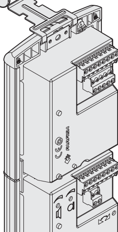
Accrocher la partie inférieure du cadre porte modules au boîtier antipluie effectuer les branchements électriques.
