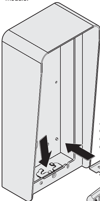
Assemblage des modules au cadre porte module.
